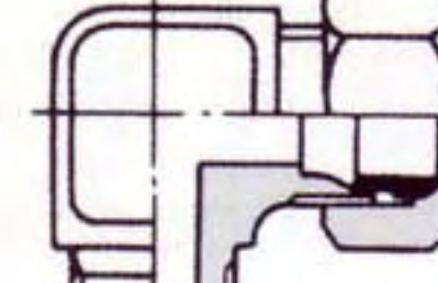
GLF EGS:ホース接続 ユニオンエルボ (めす)
