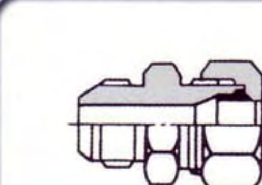
GUC UG:ホース接続ユニオン
