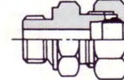
URG :平行ねじニップル (銅バスケット用)
