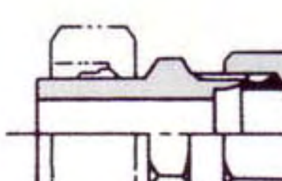
GR UPP:レジュサー
