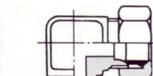
GLC EG:ホース接続ユニオンエルボ
