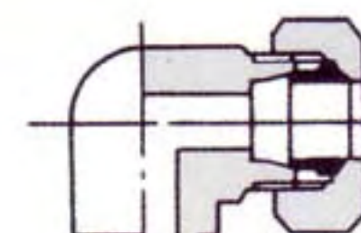
UE :方向調整型エルボニップル
