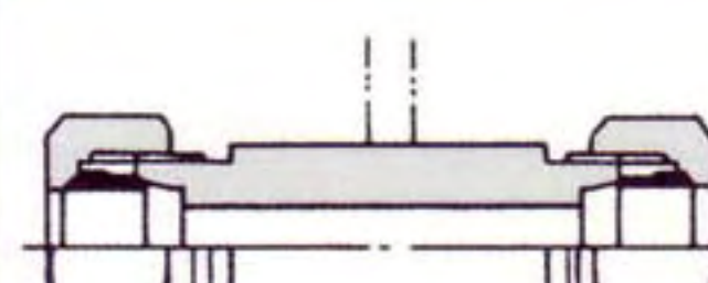
UL :隔壁溶接ユニオン
