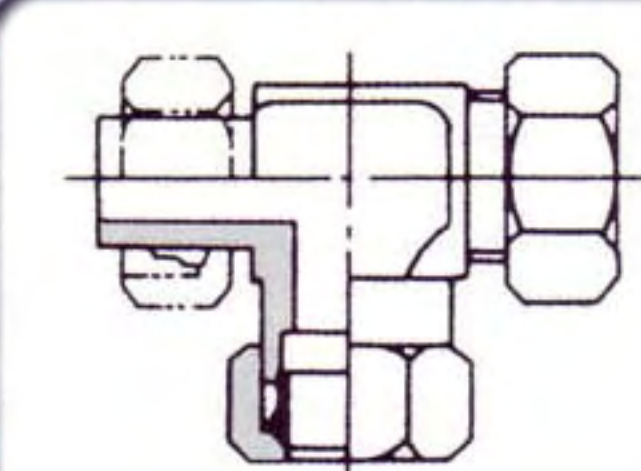
TLPP :方向調整片ティー
