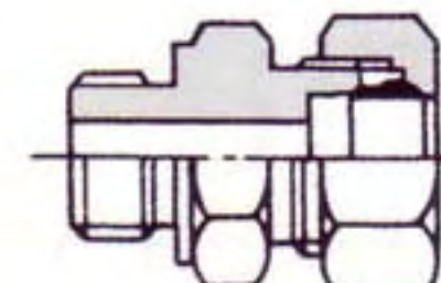
UR :平行ねじニップル (Oリング用)
